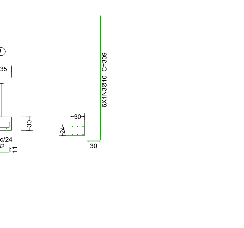
S20 Esc. 1:50
