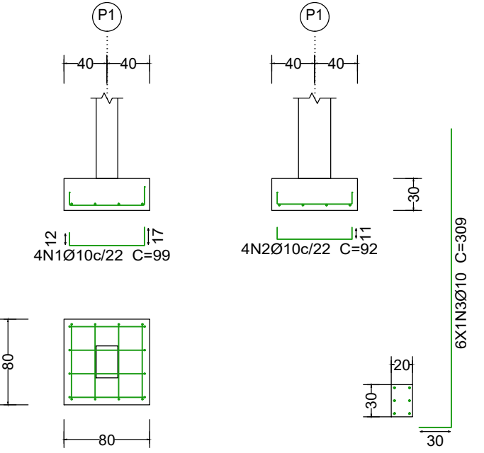
S6 Esc. 1:50
