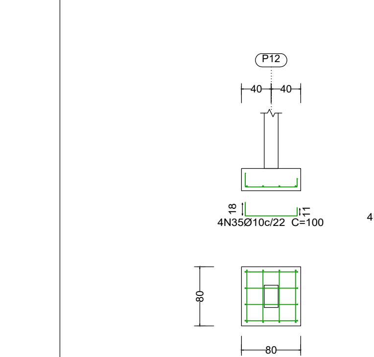
S12 Esc. 1:50
