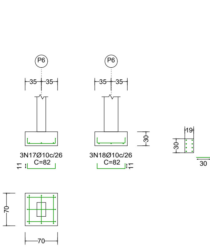
S6 Esc. 1:50
