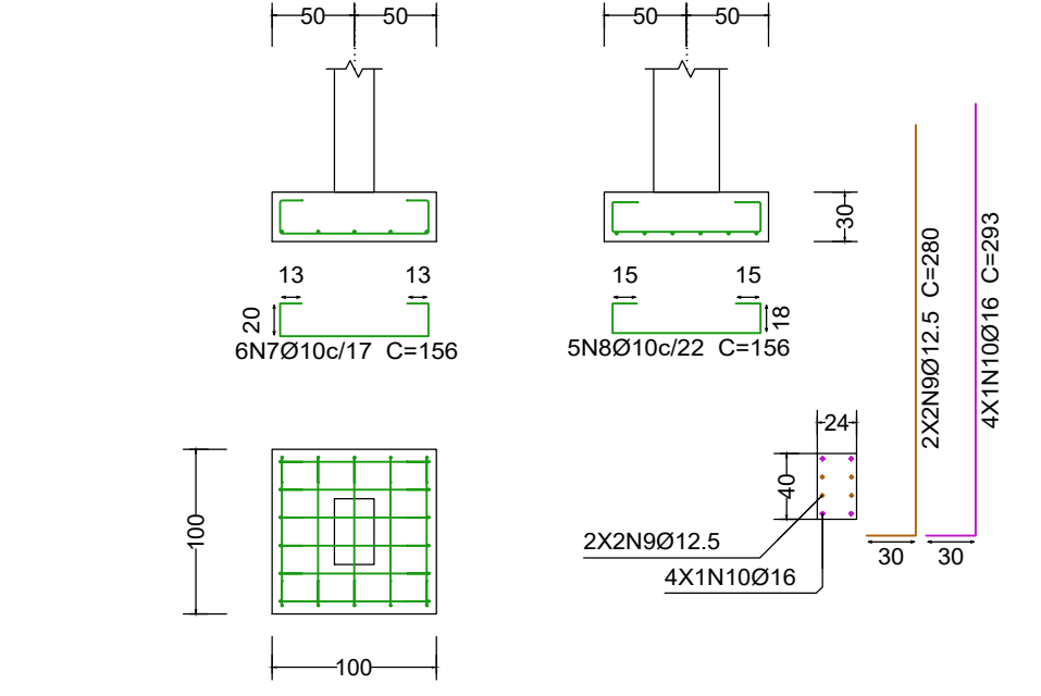
S8 Esc. 1:50
