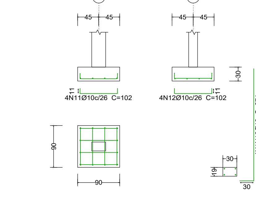
S9 Esc. 1:50
