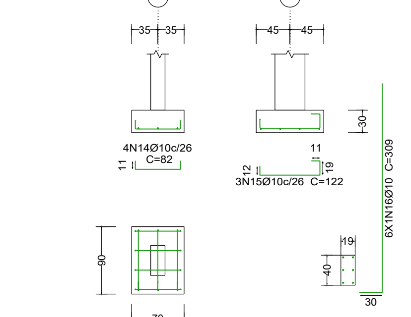
S10 Esc. 1:50
