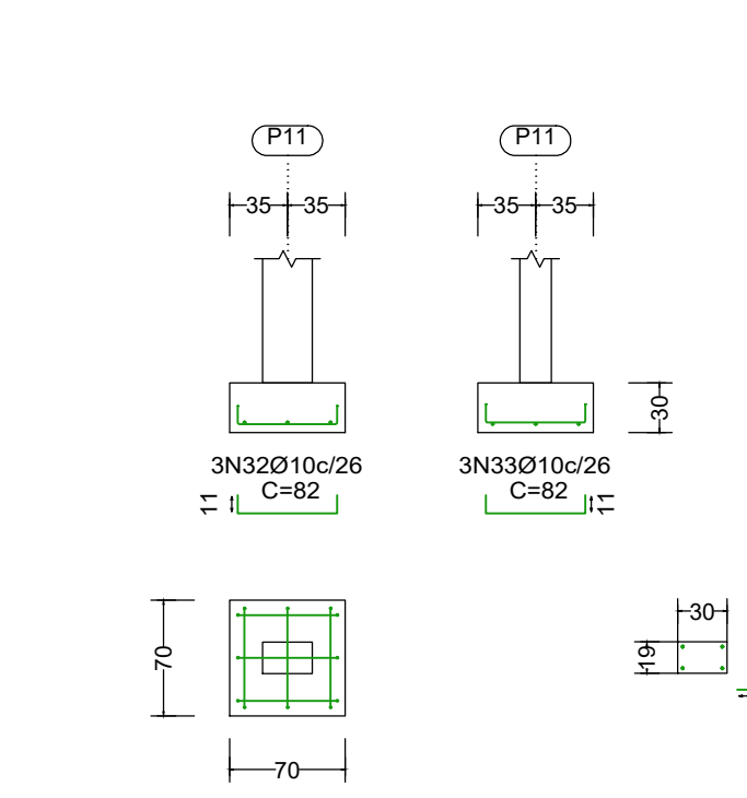
S11 Esc. 1:50
