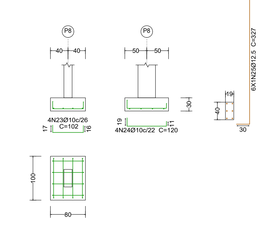
S8 Esc. 1:50
