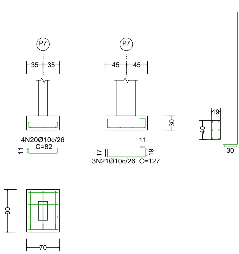
S7 Esc. 1:50
