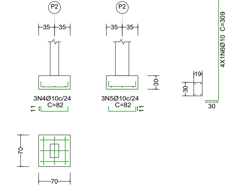
S7 Esc. 1:50
