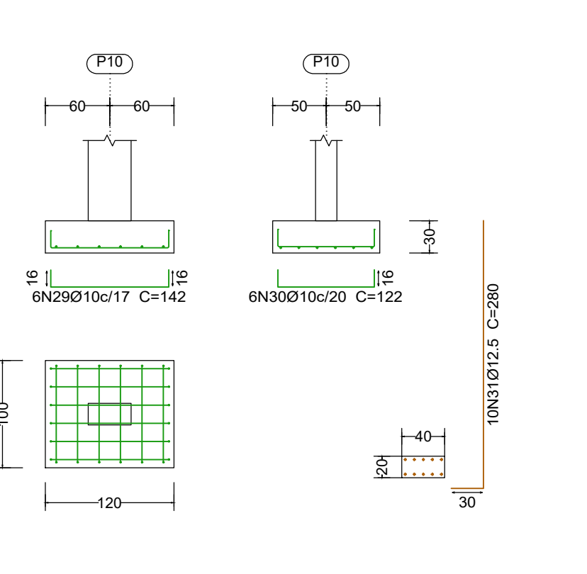
S10 Esc. 1:50
