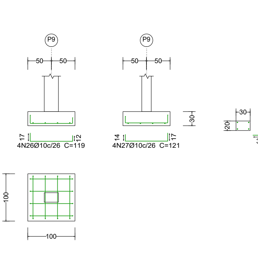
S9 Esc. 1:50
